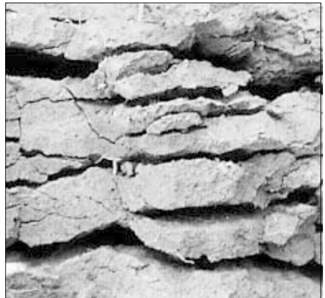
Fig. 25 : Ce sont surtout les sols silteux qui présentent une structure en feuillets, avec des fentes horizontales.
