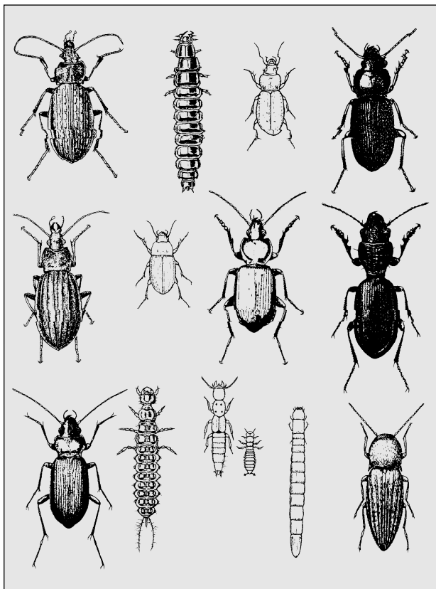
Chap. 2 Fig. 12 : Carabes avec leur larve (Taille entre 7 et 33 mm).
